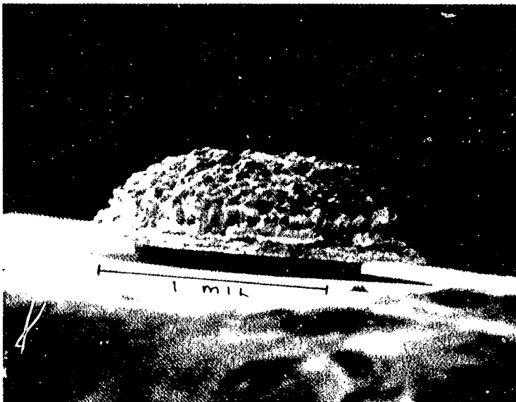
Fig. 21—IMPATT diode.
