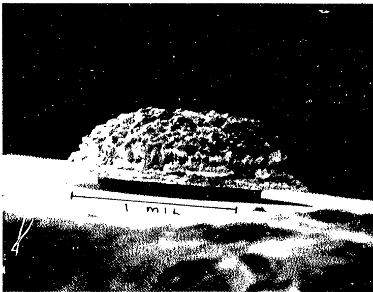
Fig. 21—IMPATT diode.
